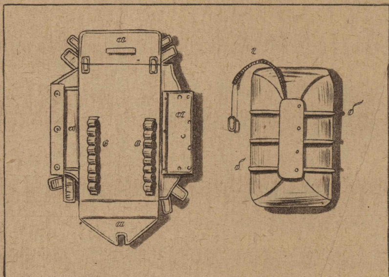
Парашют Гюи Болла фирмы «Ирвин Эйршют К о » 1925 года: а — клапаны; б — резинки; в — соты; г — строенная тросовая шпилька.
