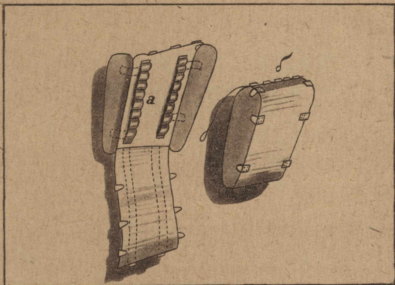
Ранец парашюта «РК-2» с сотами для строп и строенной тросовой шпилькой: а — соты, б — шпилька.
