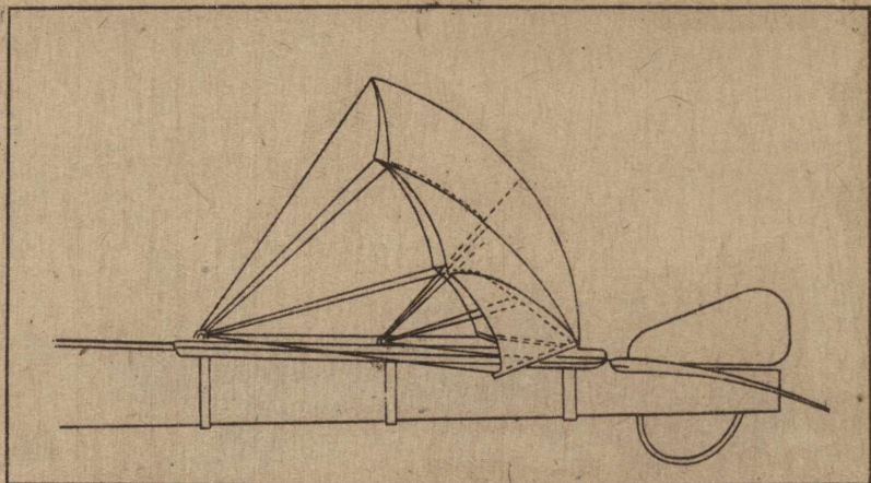
Парашютный тормоз 1912 года конструкции Г. Котельникова. (По чертежу автора.)
