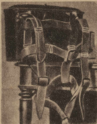
Ранцевый парашют «РК-1» образца 1914 года. (Фото автора.)
